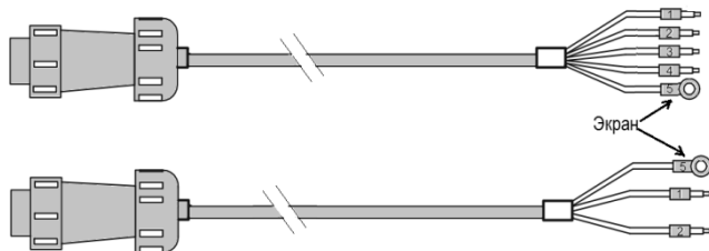
Рисунок Л3 Внешние кабели ПРЭМ
