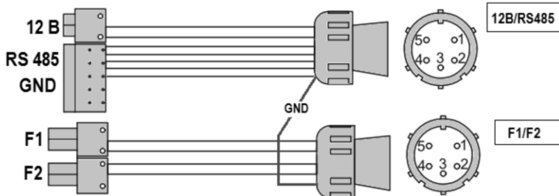
Рисунок Л1 Внутренний шлейф ПРЭМ
