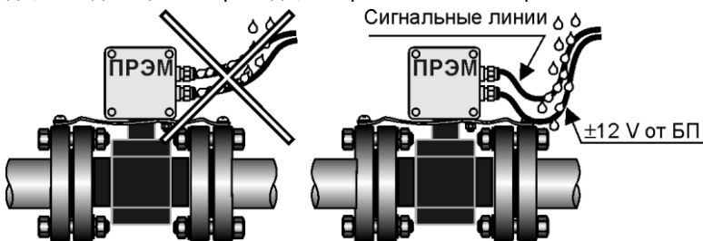
Рисунок 22 – Прокладка кабелей
