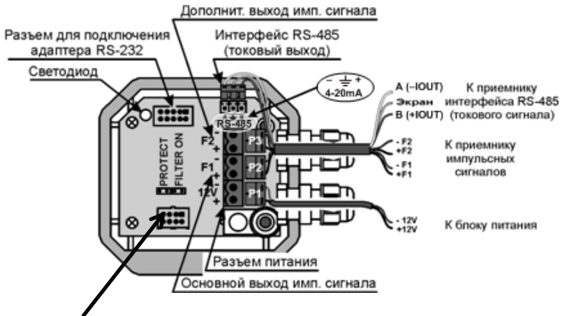
Разъём подключения катушек
