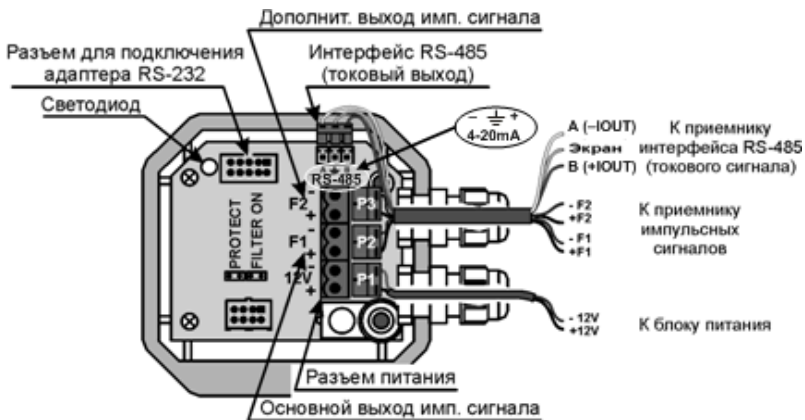
Рисунок 21 – Схема расположения клеммников на примере платы P542_1352
