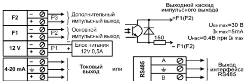
Рисунок 20 – Схема подключения ПРЭМ P542_1352
