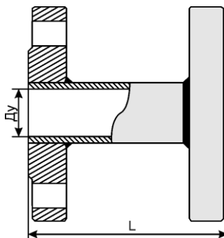
Габаритный имитатор ИПФ Для ПРЭМ фланцевого исполнения
