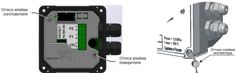
Рис. 4 – Места пломбирования
