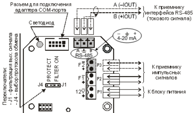
Рис. 2 - Внешний вид платы блока электронного преобразователя P542_1352
