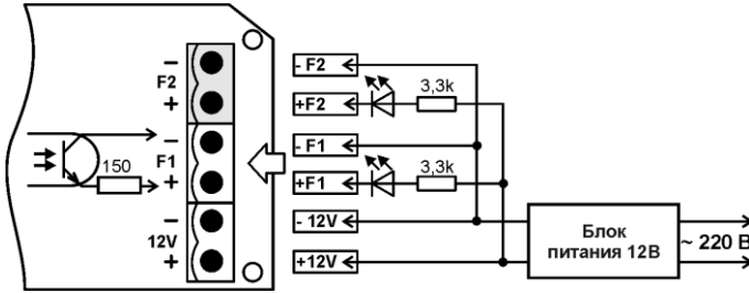
Рисунок 23 – Контроль выходных сигналов P542_1352
