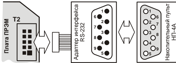
Рисунок И.2 – Схема подключения к НП-4 через внешний интерфейс RS-232
