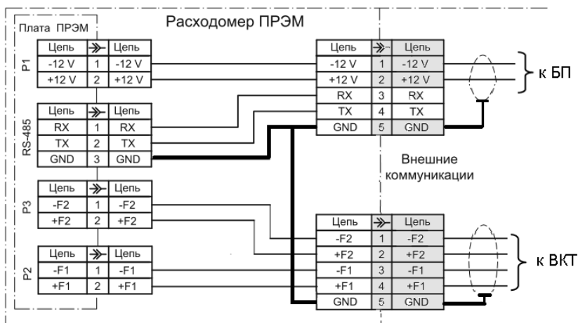
Рисунок Л2 Схема распиновки «выходов» из ПРЭМ
