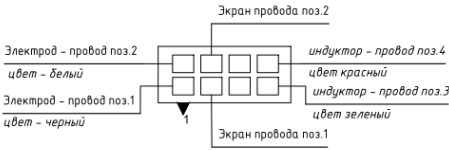
Рисунок М3 Разъём подключения катушек
